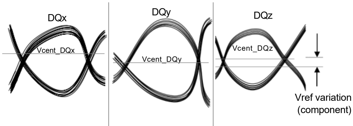
Figure 8-9 Across Pin Vref DQ Voltage Variation
